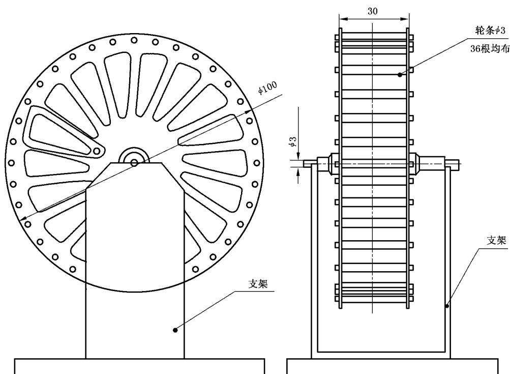
图 3 小鼠转笼
