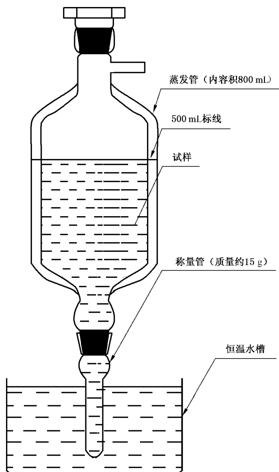
图 1 蒸发器
